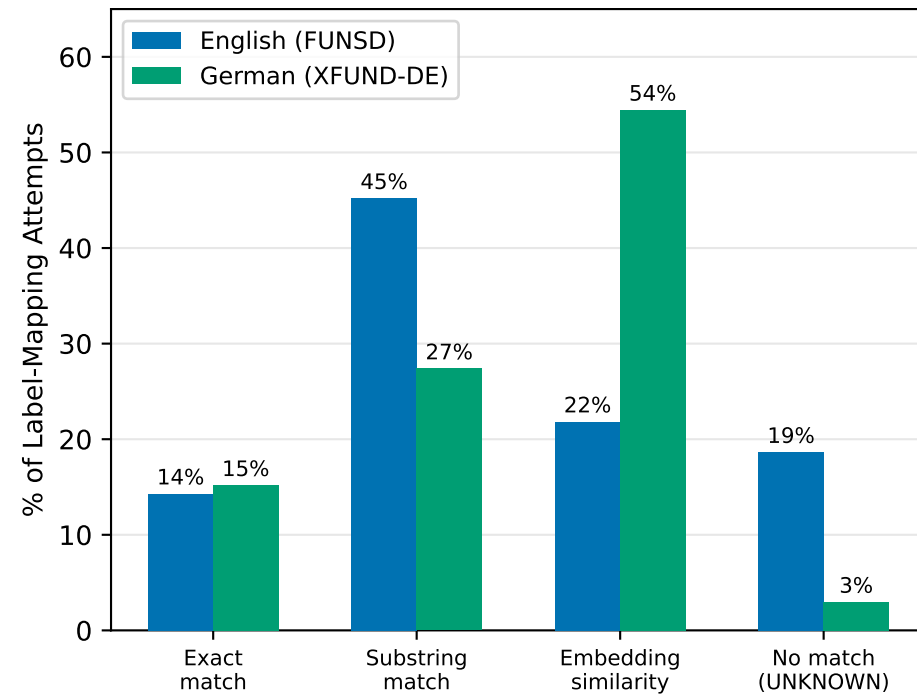
Label Resolution Phase Distribution EN vs DE
