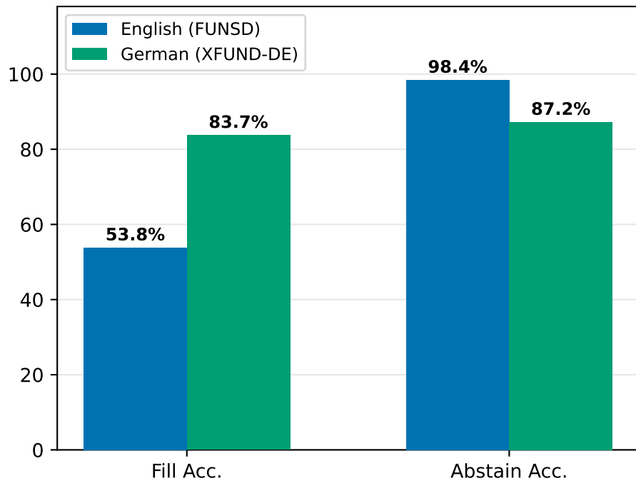
Fill & Abstain Accuracy EN vs DE
