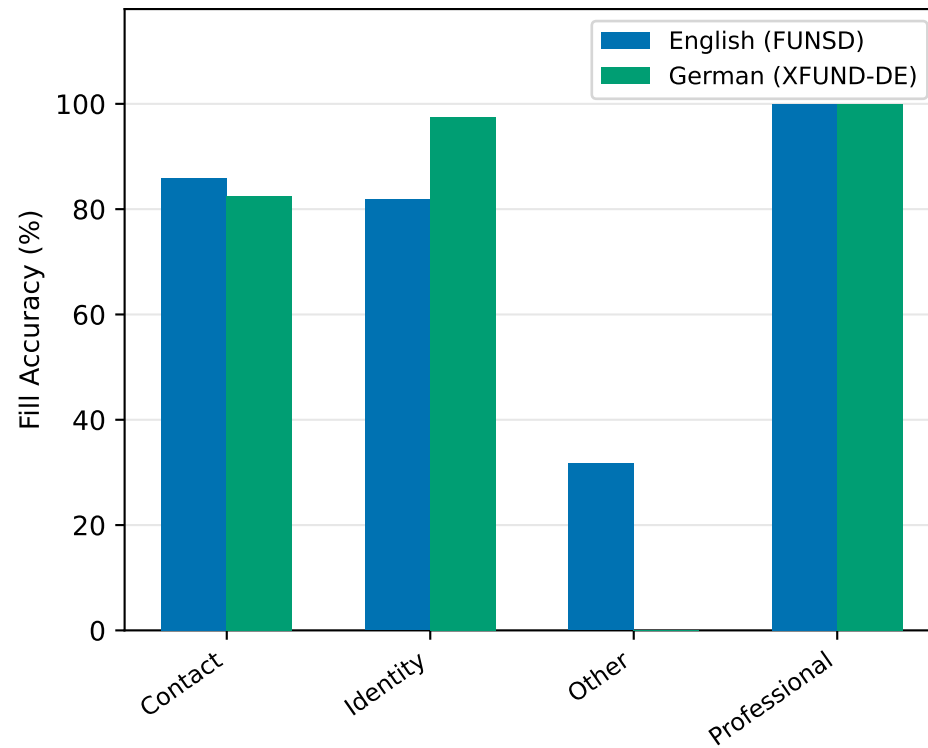
Per-Category Fill Accuracy EN vs DE
